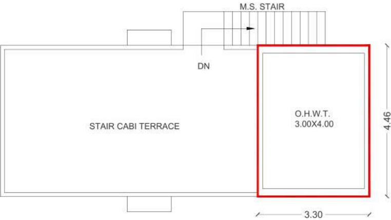
O.H.W.T. PLAN
