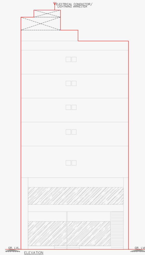
ELEVATION
