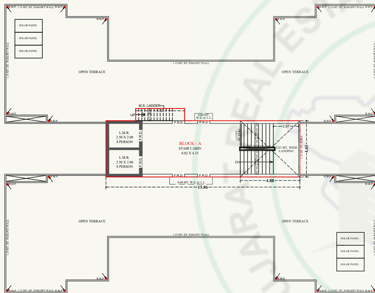
OPEN TERRACE PLAN (STAIR CABIN & O.H.W.T.)
