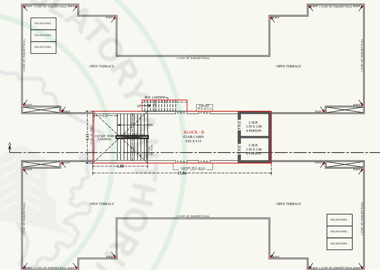
OPEN TERRACE PLAN (STAIR CABIN & O.H.W.T.)
