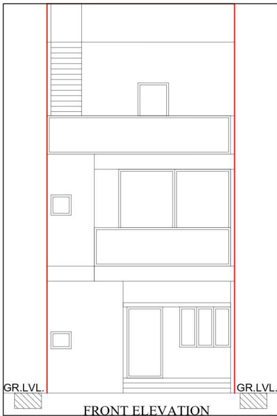
ELEVATION
