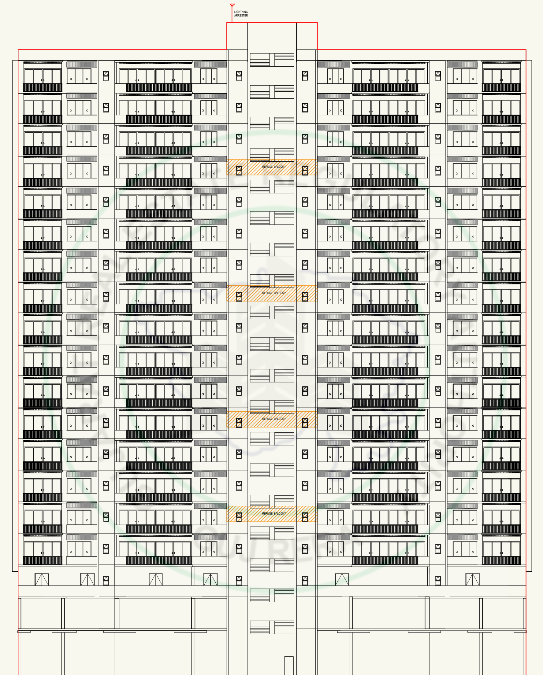
ELEVATION
