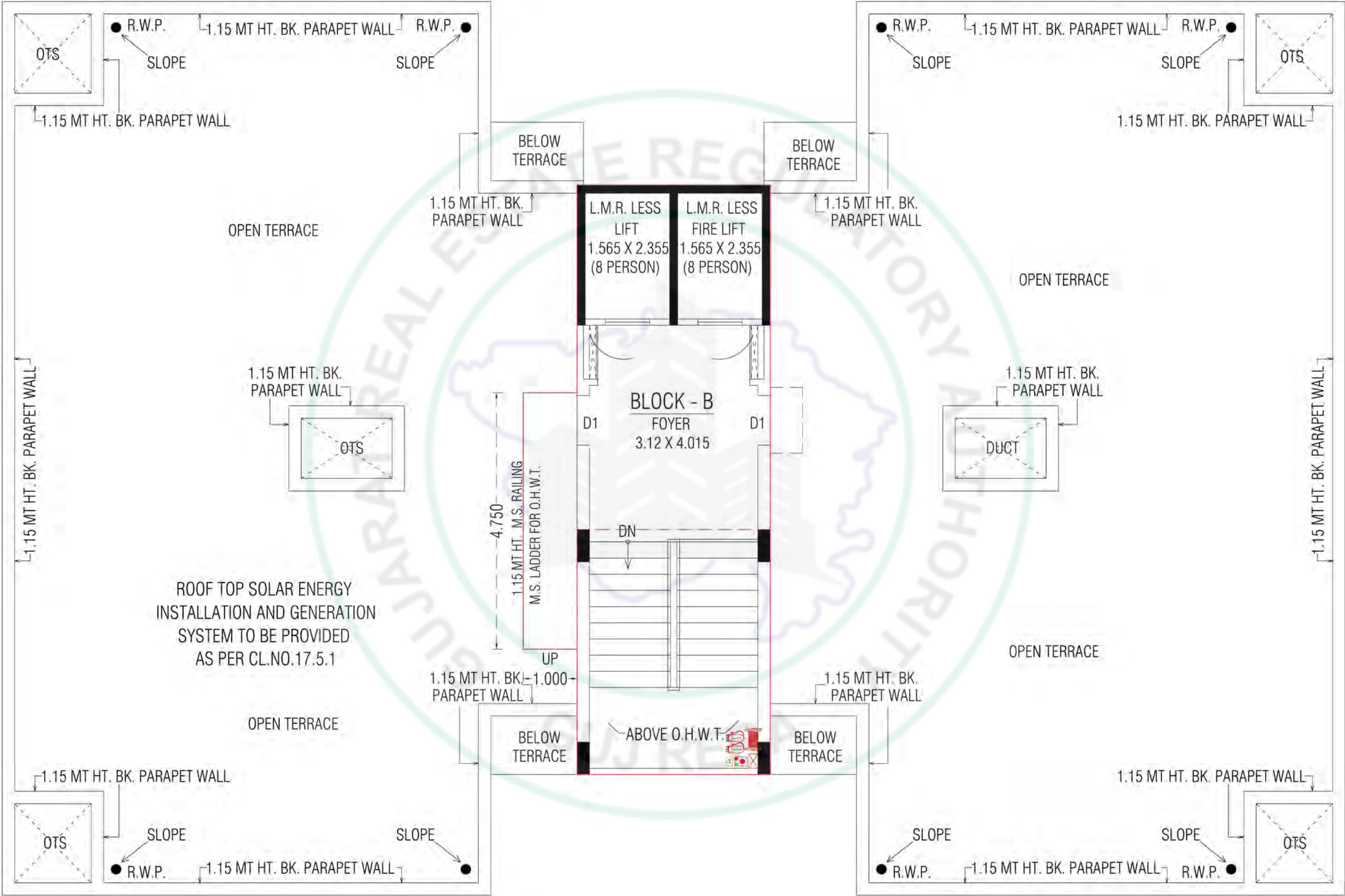
STAIR CABIN , O.H.W.T. & OPEN TERRACE PLAN
