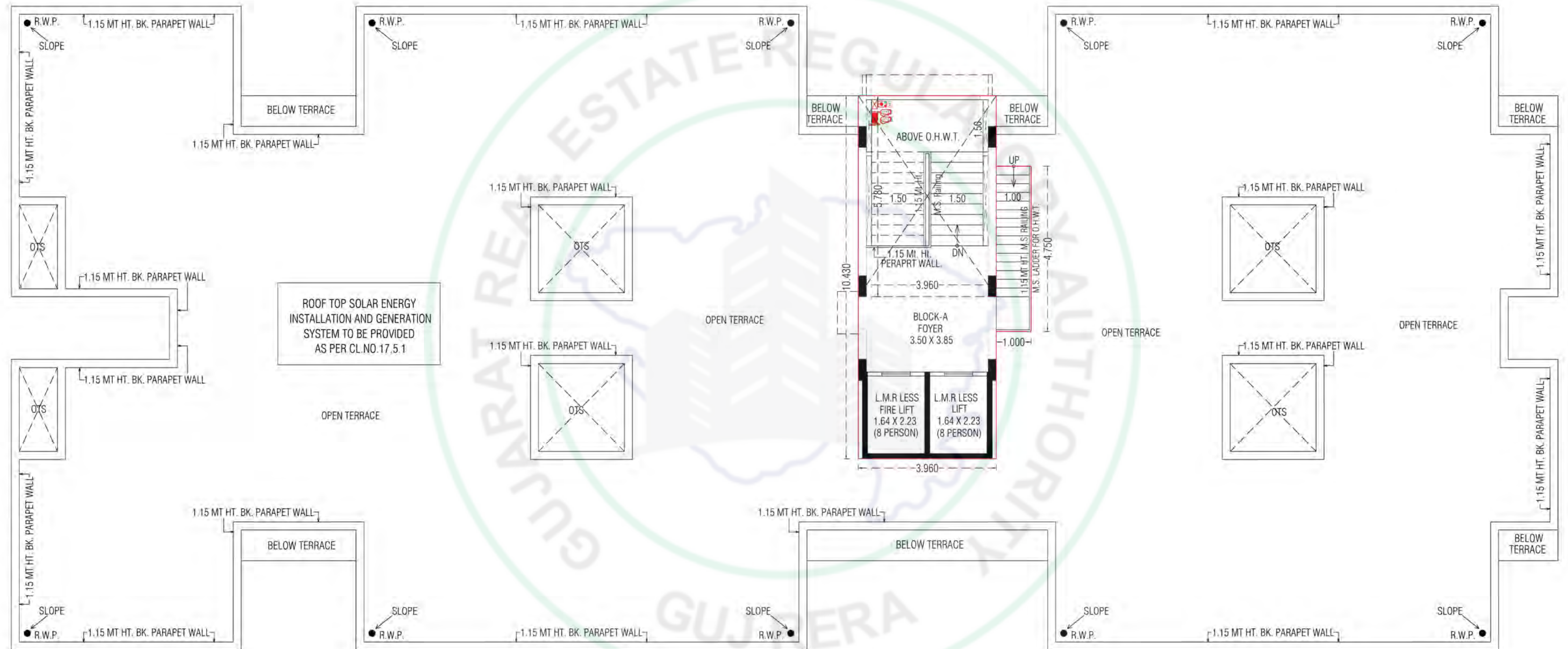
STAIR CABIN , O.H.W.T. & OPEN TERRACE PLAN
