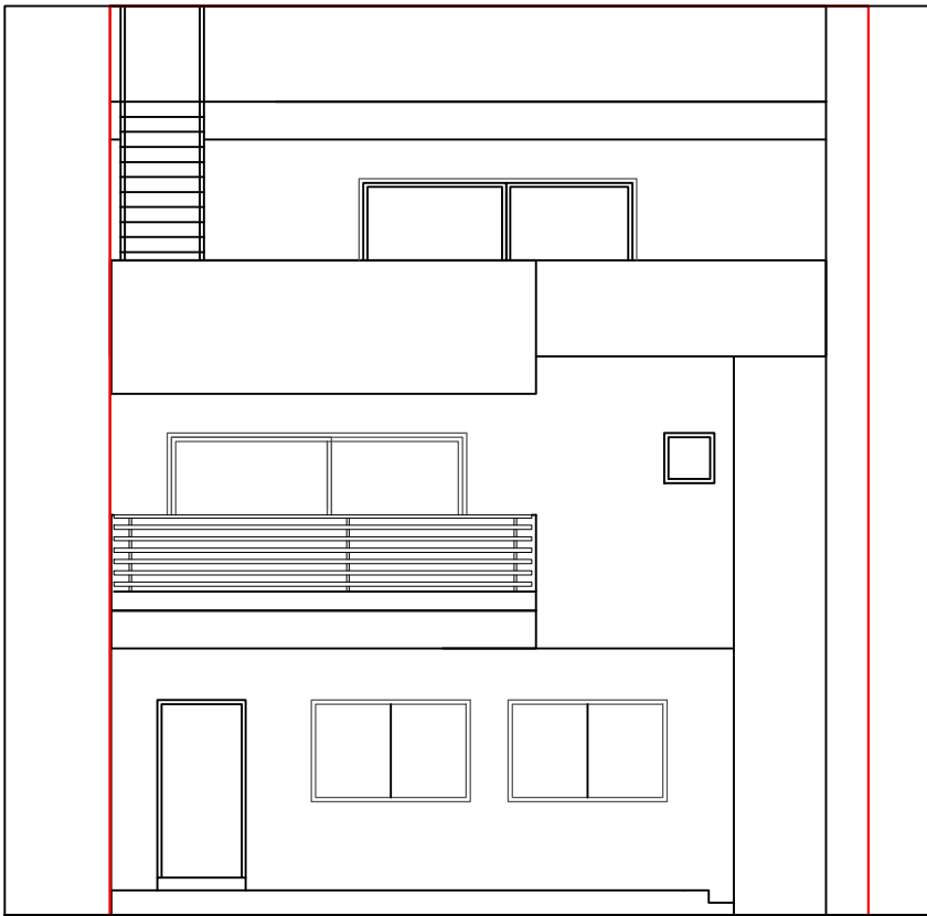
ELEVATION
