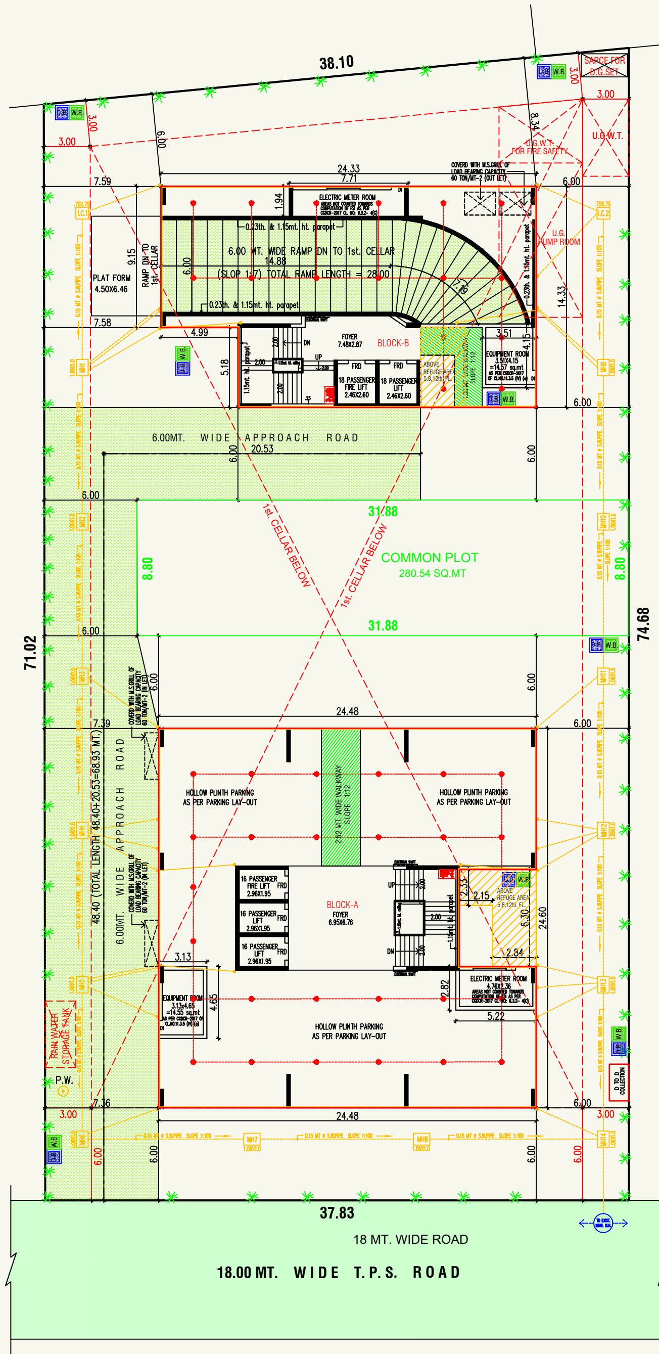
LAY-OUT PLAN
