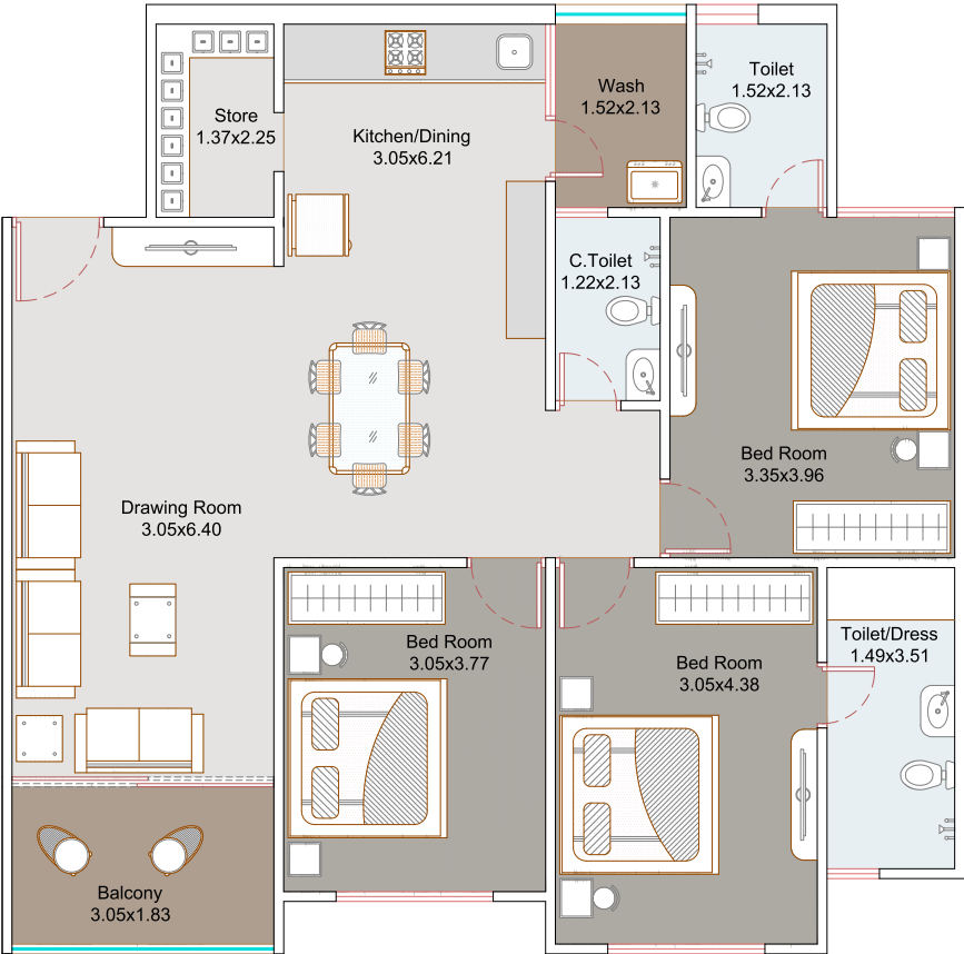
C 201 - 1401
