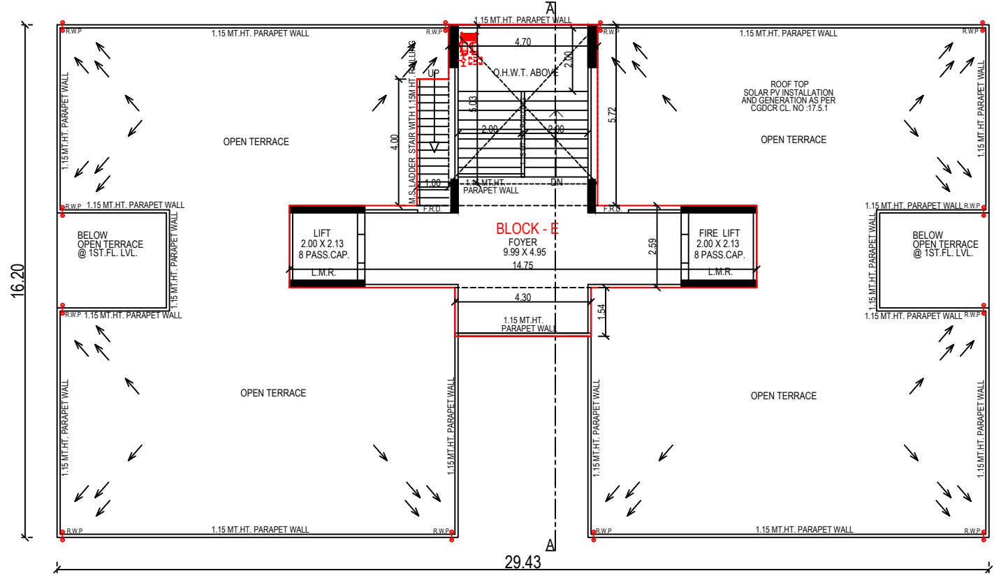
OPEN TERRACE , STAIR CABIN, LMR. & O.H.W.T. PLAN (BLOCK - E)
