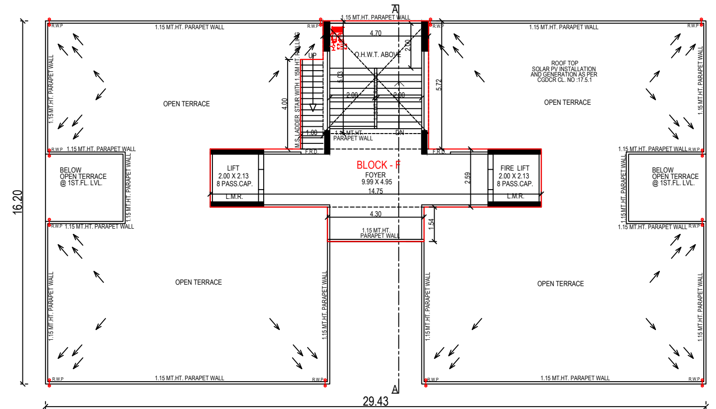
OPEN TERRACE , STAIR CABIN, LMR. & O.H.W.T. PLAN (BLOCK - F)
